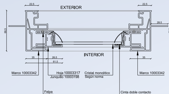
Detalle 2
