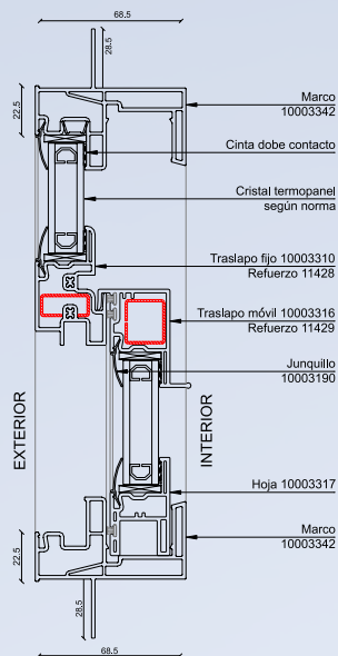
Detalle 1
