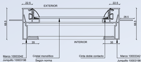
Detalle 2
