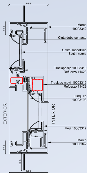
Detalle 1
